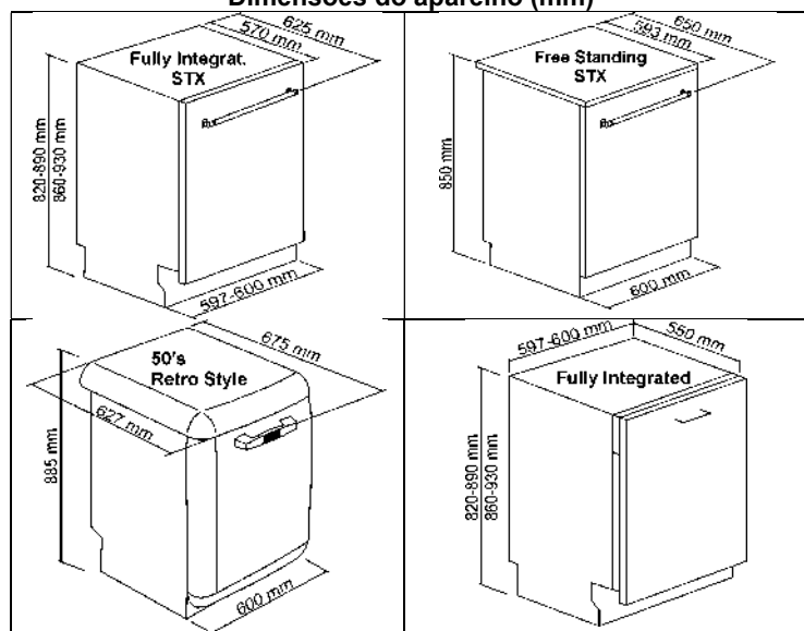
Dimensões do aparelho (mm)
