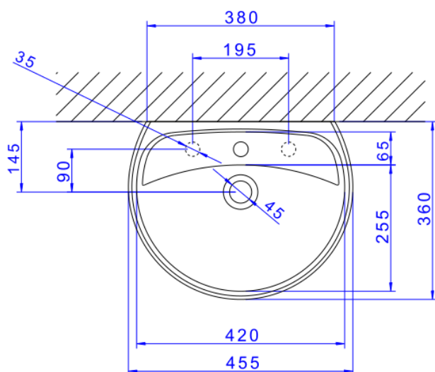
Desenho Técnico
