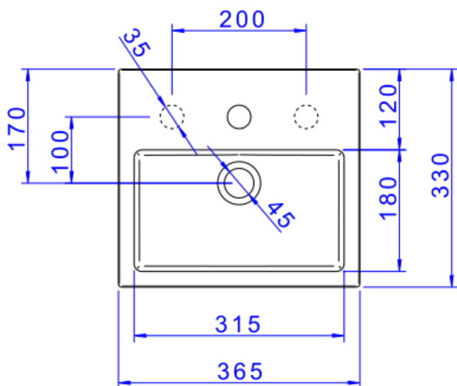
Desenho Técnico
