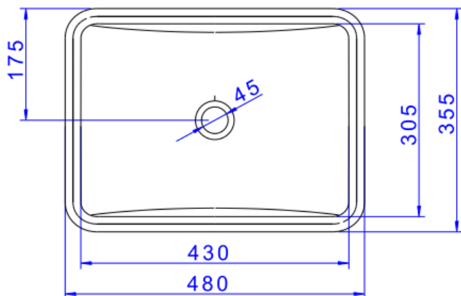
Desenho Técnico
