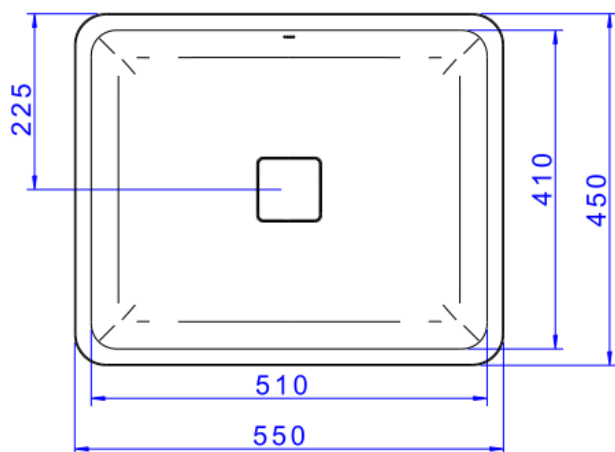
Desenho Técnico
