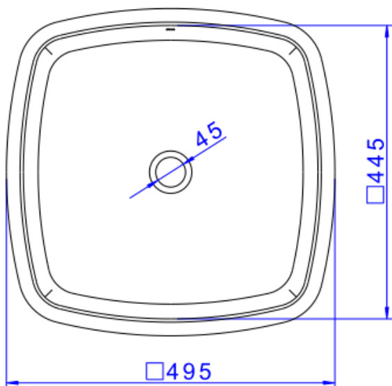
Desenho Técnico
