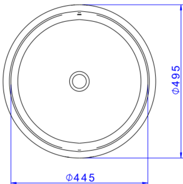
Desenho Técnico
