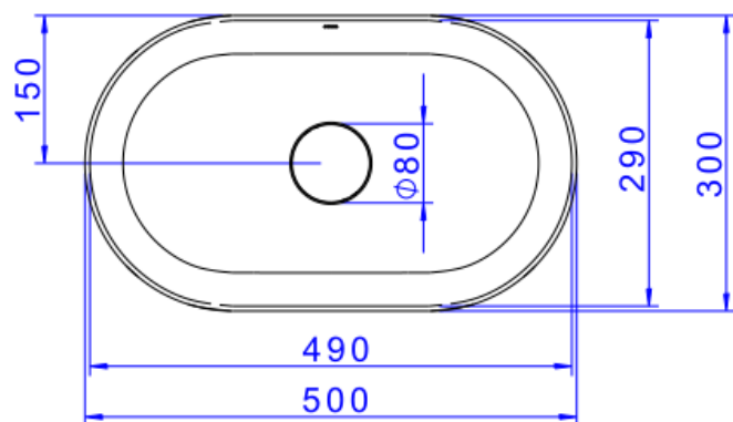
Desenho Técnico
