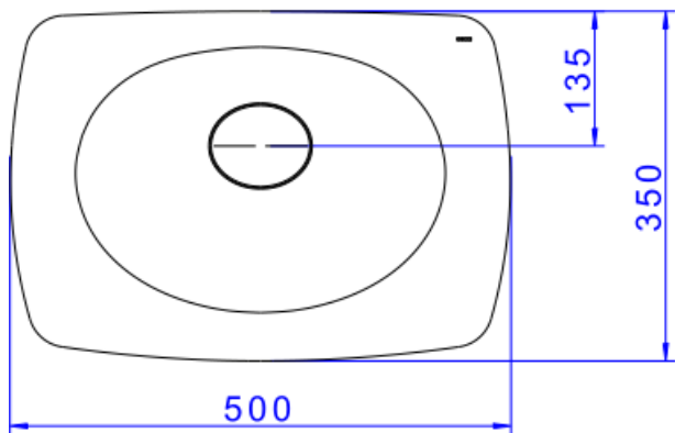
Desenho Técnico
