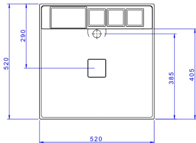
Desenho Técnico
