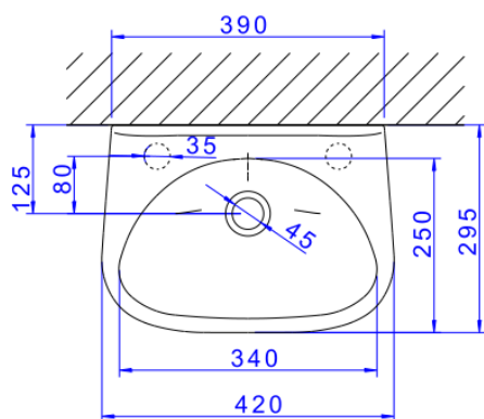
Desenho Técnico
