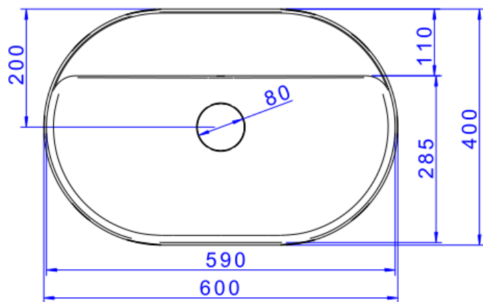
Desenho Técnico
