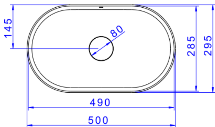
Desenho Técnico
