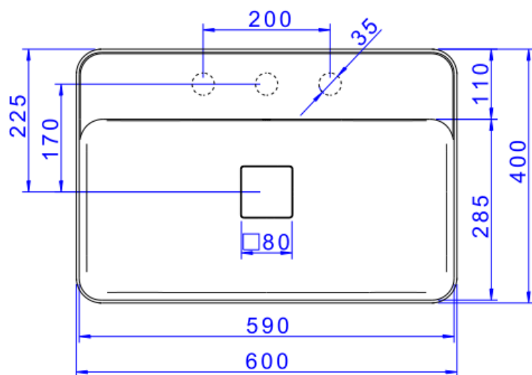
Desenho Técnico
