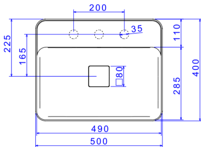
Desenho Técnico
