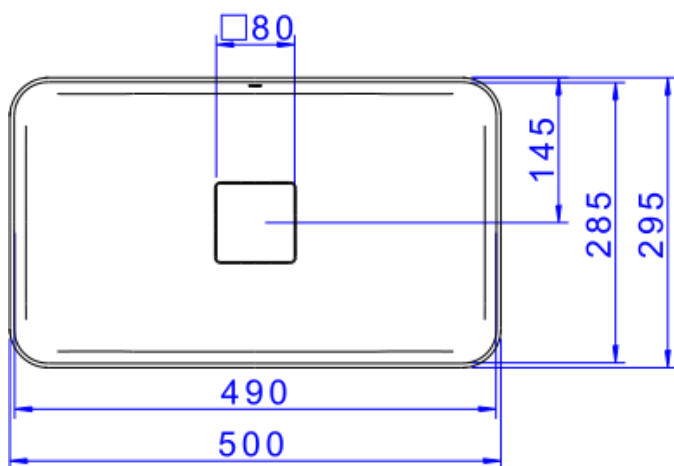
Desenho Técnico
