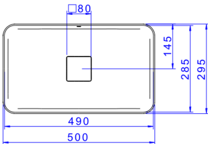
Desenho Técnico
