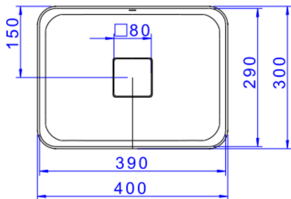
Desenho Técnico
