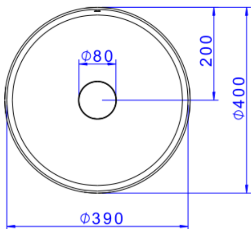
Desenho Técnico
