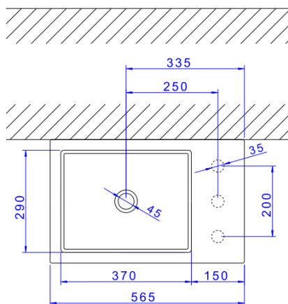
Desenho Técnico
