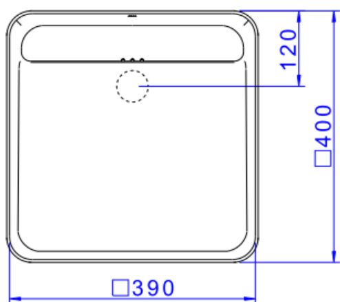
Desenho Técnico
