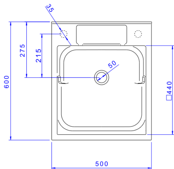
Desenho Técnico
