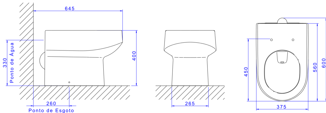
Desenho Técnico
