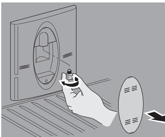
Lâmpadas do congelador
