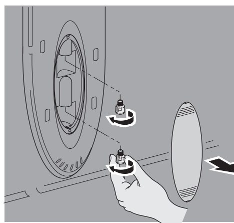
Lâmpadas do frigorífico
