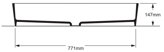
Vista lateral
