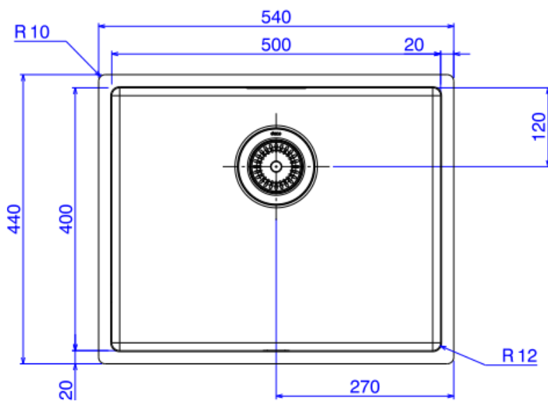
Desenho Técnico
