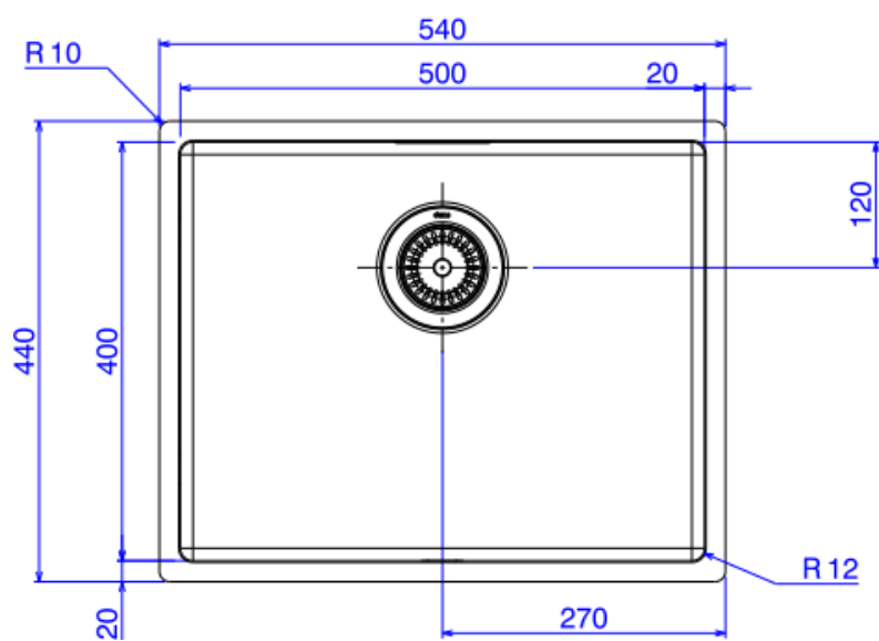
Desenho Técnico
