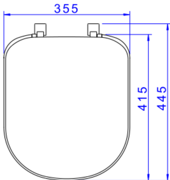
Desenho Técnico
