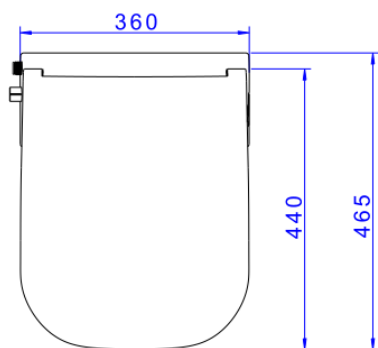
Desenho Técnico
