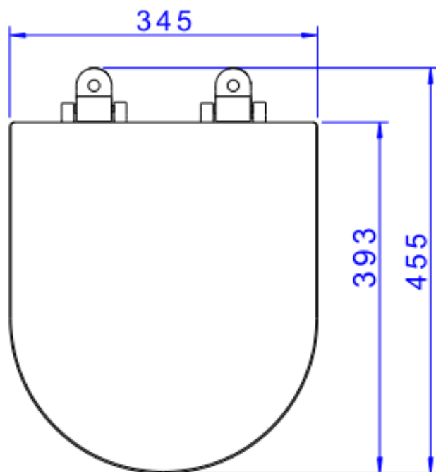
Desenho Técnico
