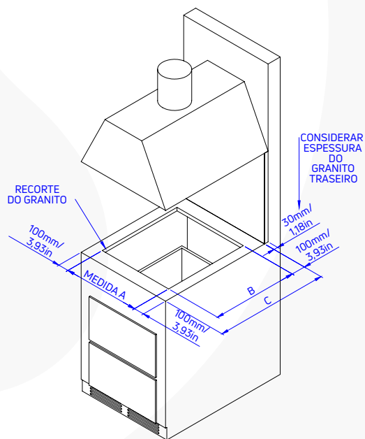
VISTA PROJETADA
