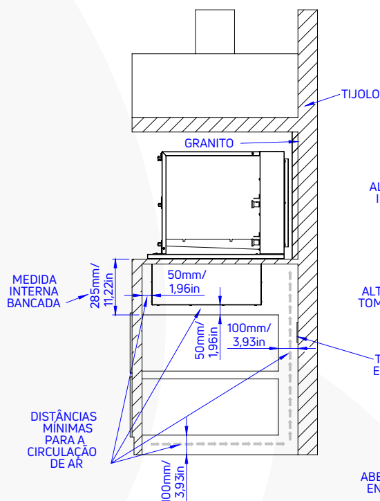
Seção A
