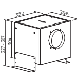
Instalação horizontal do motor
