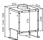
Instalação vertical do motor
