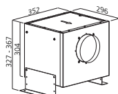
Instalação horizontal do motor
