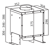
Instalação vertical do motor
