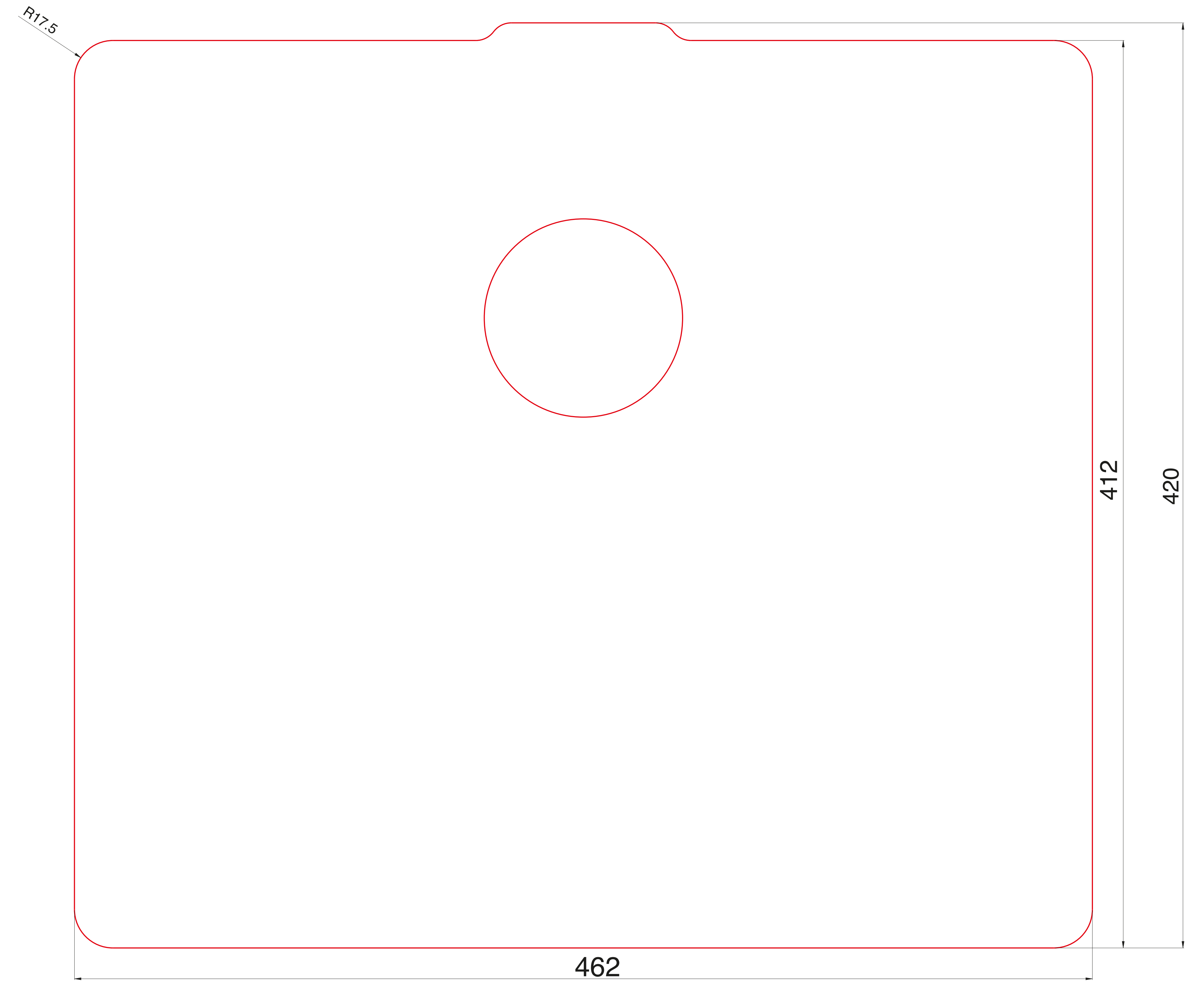
Dimensões para desenvolvimento da faca de corte
