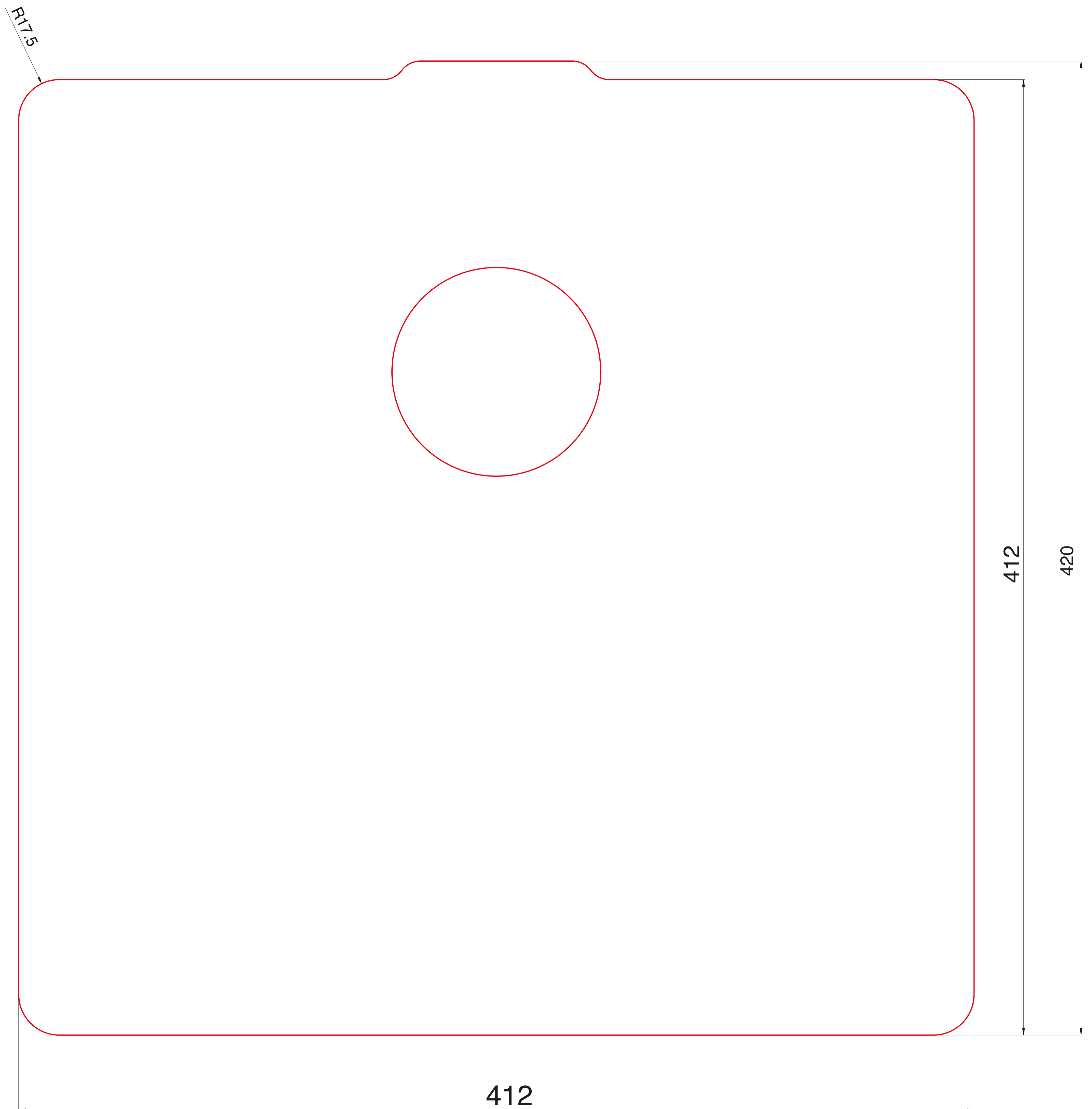
Dimensões para desenvolvimento da faca de corte
