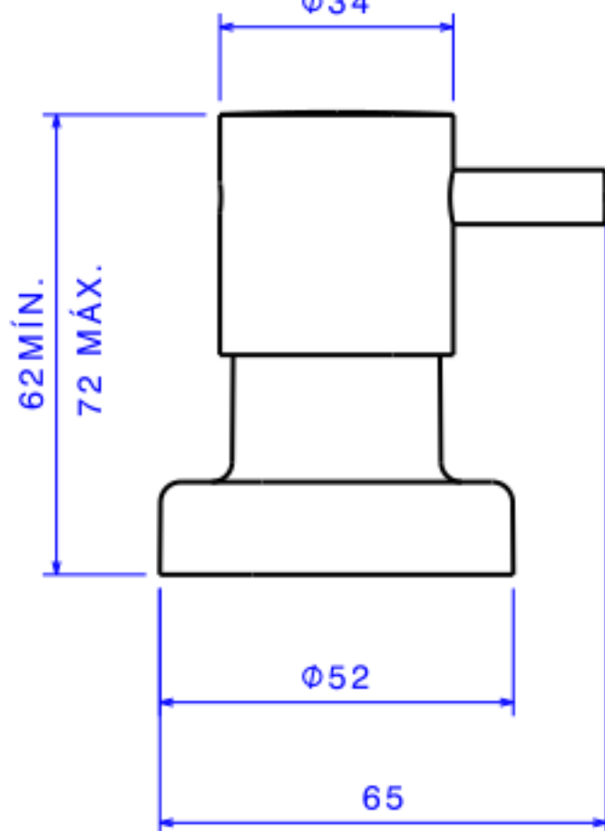
Desenho Técnico
