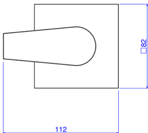
Desenho Técnico
