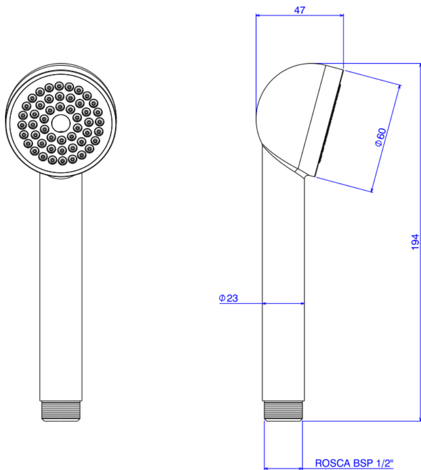
Desenho Técnico
