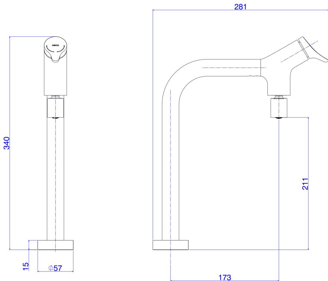
Desenho Técnico
