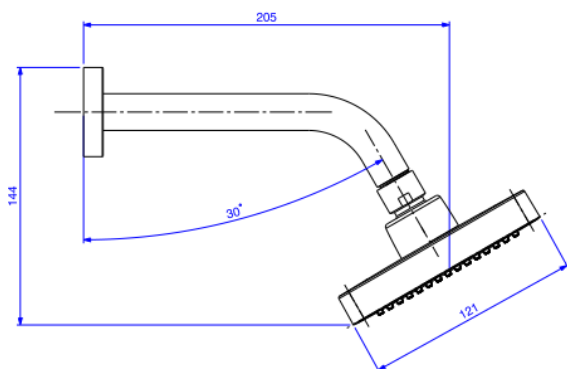
Desenho Técnico
