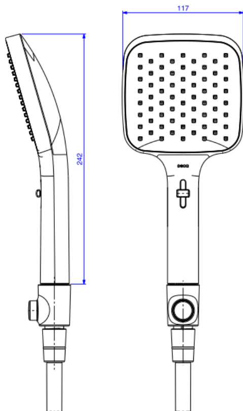
Desenho Técnico
