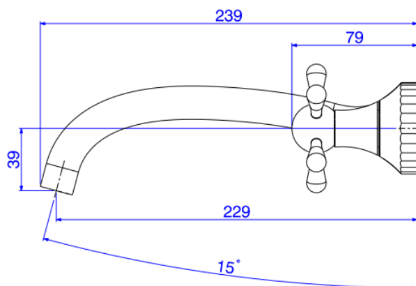
Desenho Técnico
