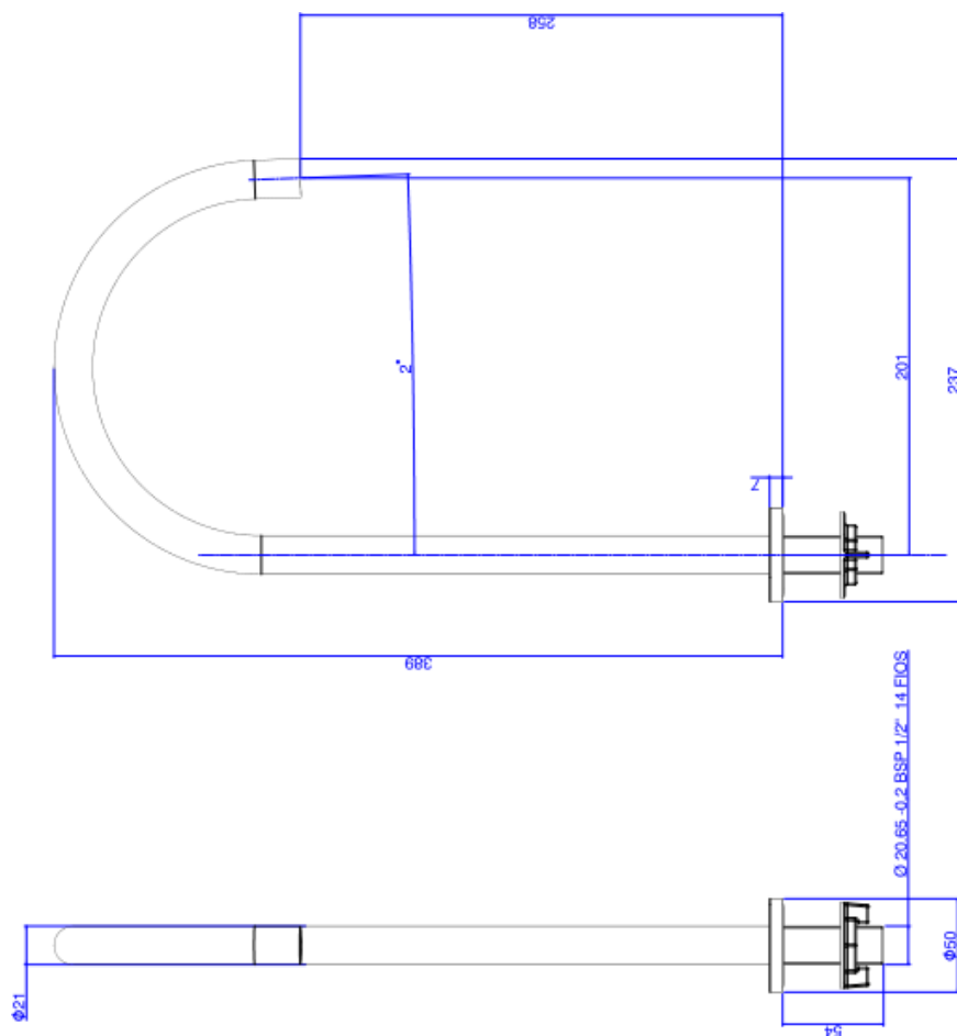
Desenho Técnico
