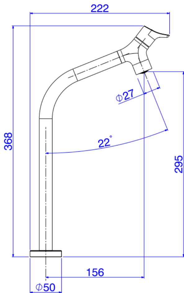
Desenho Técnico
