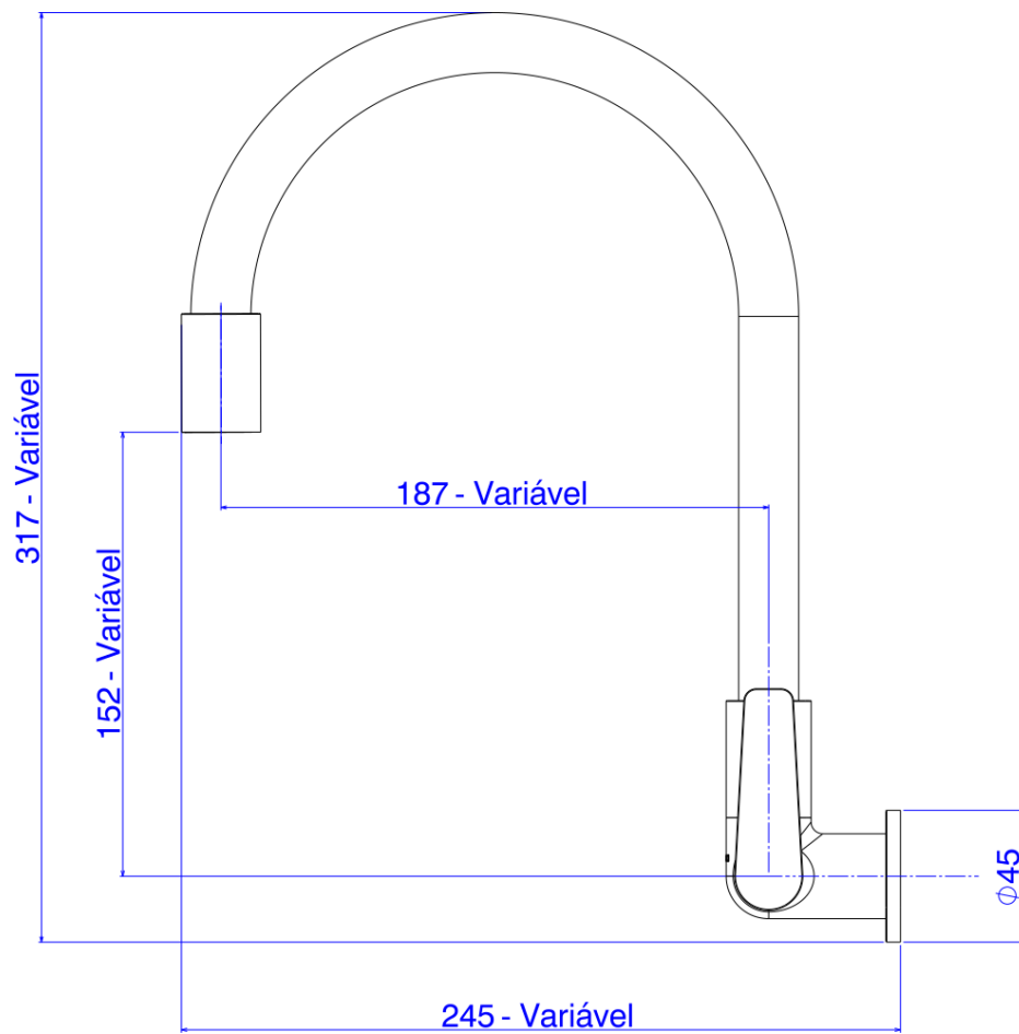
Desenho Técnico
