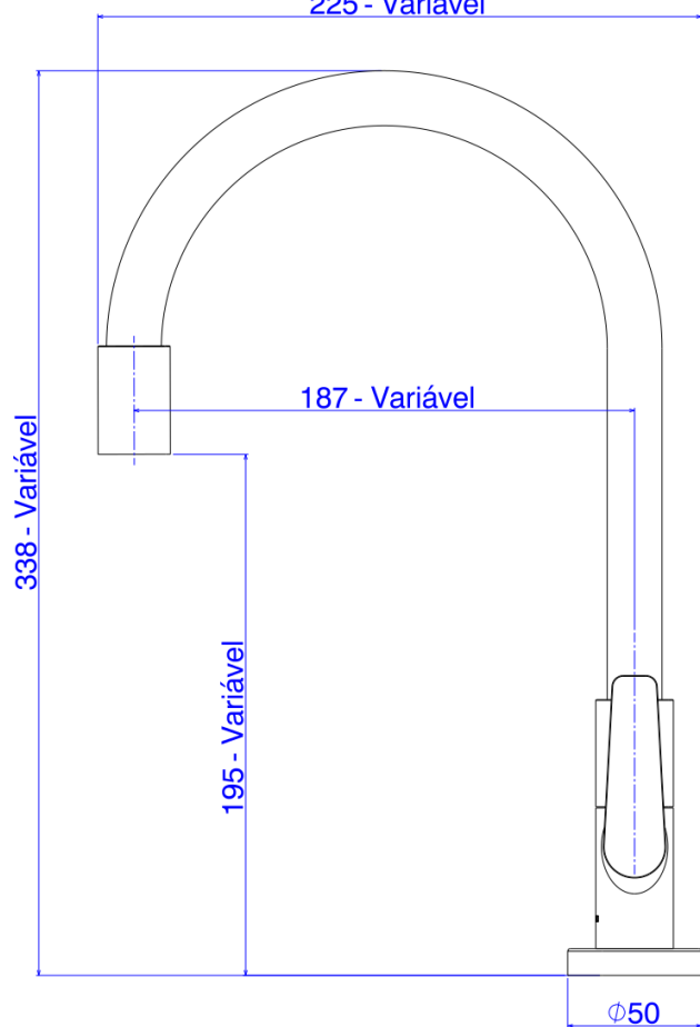
Desenho Técnico
